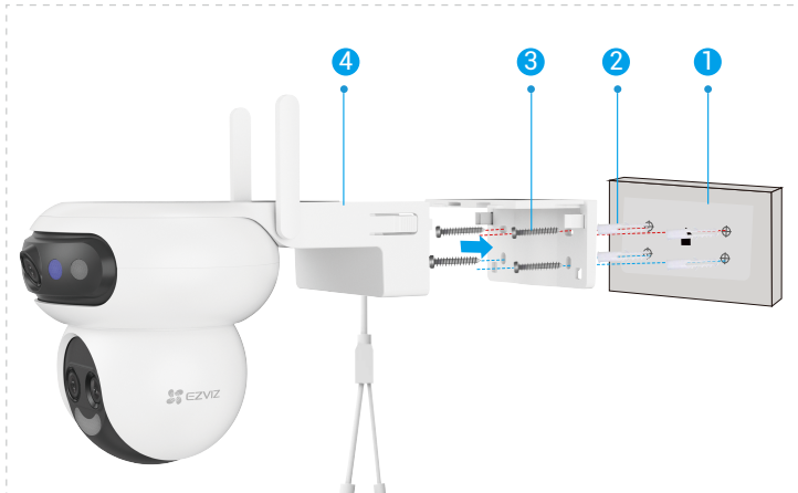
圖 2 壁掛式安裝
